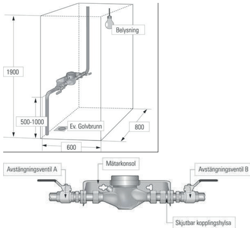
Figur 2: exempel på godkänd vattenmätarkonsol med avstängningsventiler.
